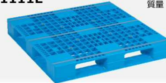
AZFD-1210E サイズ: 1200×1000×150Hmm 質量: 13.7kg
